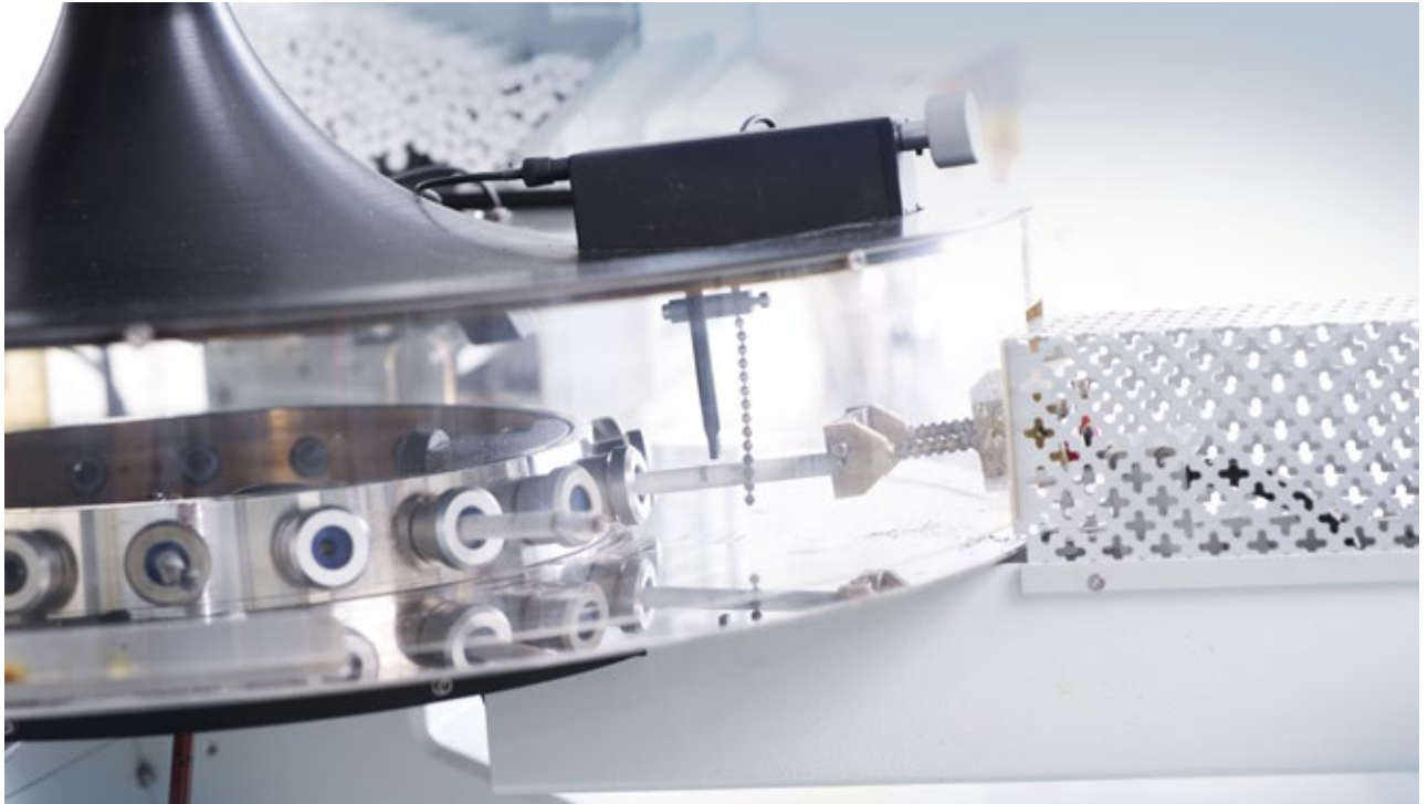
Vorrichtung zur Produktion von kontrolliertem Zigarettenrauch für experimentelle Modelle.
